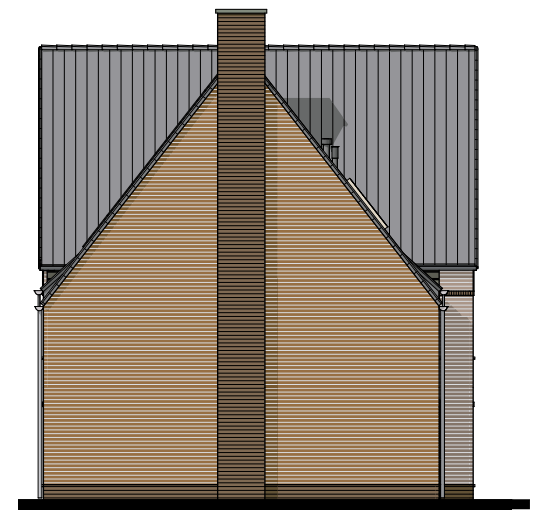
Zijgevel bnr. 31
