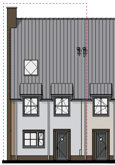
bnr. 47 Voorgevel
